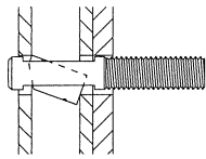
締結物が中空の場合
