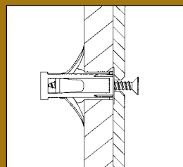
③取り付け物をセットしビスをねじ込む。
