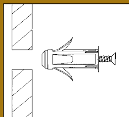
①下穴にカベアンカーを差し込む。
