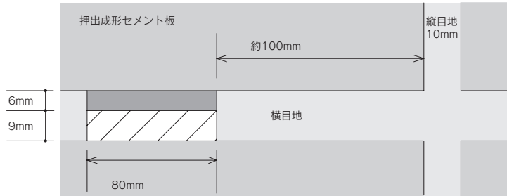
押出成形セメント板取付例
