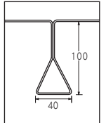
JFE建材 Hiデッキ100
