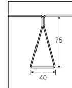
神鋼建材工業 Fデッキ
