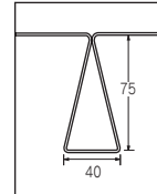
JFE日建板・北海鋼機 Fデッキ
