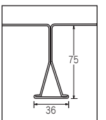
植木鋼管 Uデッキ
