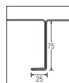
住友金属建材 Lデッキ
