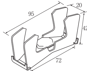
JFE建材 Nデッキ
