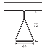
JFE建材 Nデッキ
